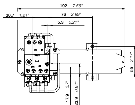
E500DU
