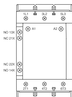
AF116 ... AF370-30-11
