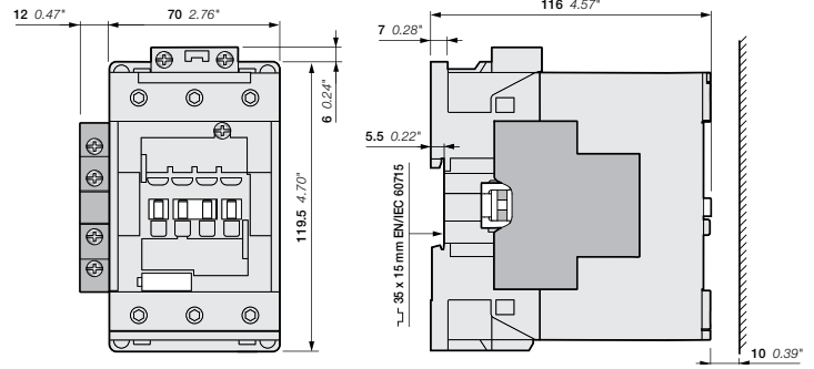
AF80N3
