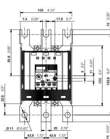
EF370-380
