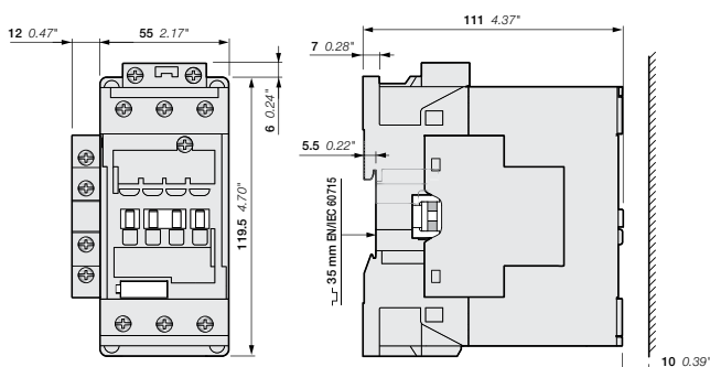
AF40N2
