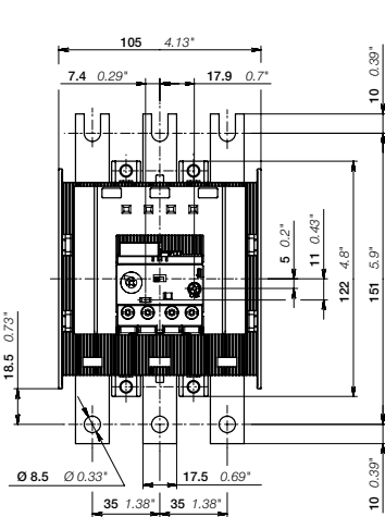
EF205-210
