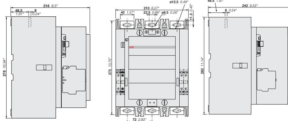
AF580, AF750
